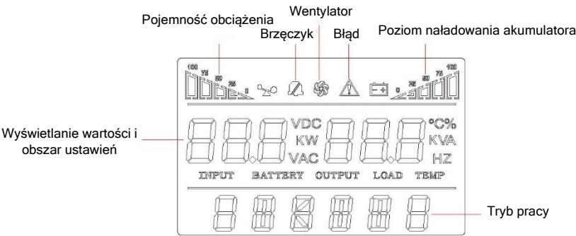
Rys. 3-2: Menu wyświetlacza
