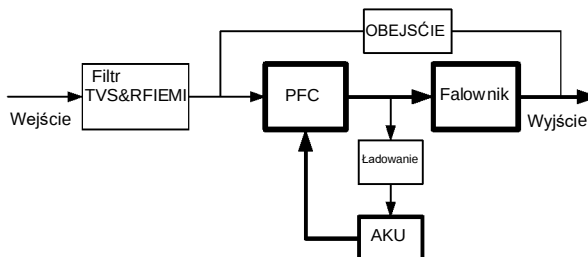
Rys. 1-6. Tryb akumulatora
