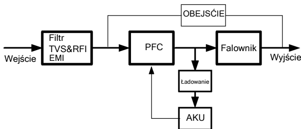
Rys. 1-4: Tryb normalny
