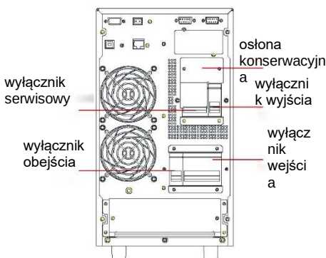
Rys. 4-1: Obejście serwisowe
