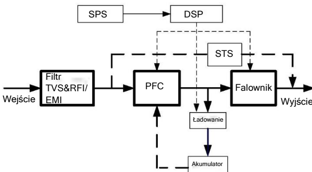
Rys. 1-3: System zasilania bezprzewodowego
